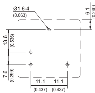
1P SPNC
