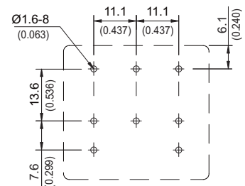
3P TPNC
