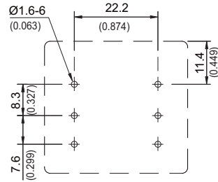
2P DPNO
