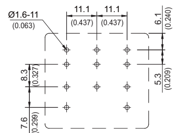
3P TPDT
