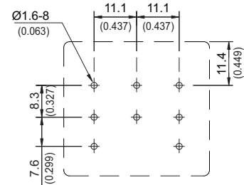
3P TPNO
