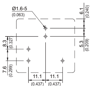
1P SPDT
