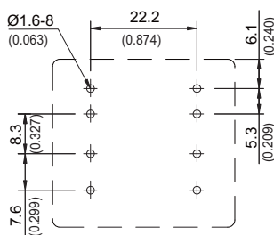
2P DPDT
