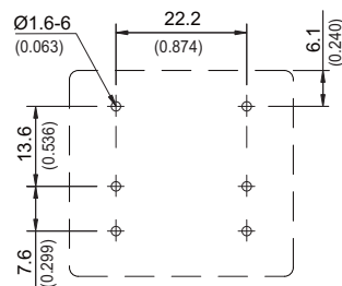
2P DPNC
