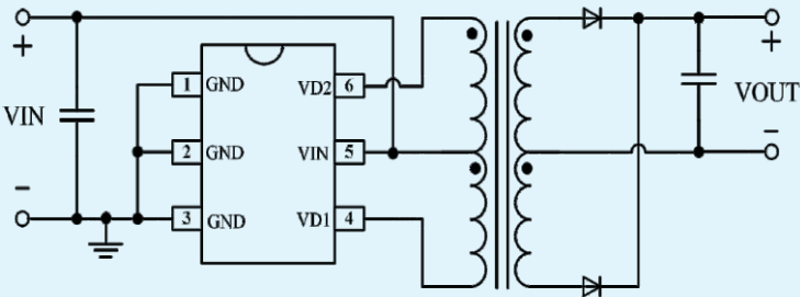
SCM1201A应用案例
