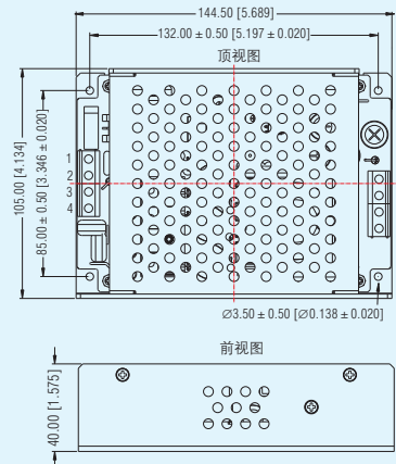
PV120-27B系列 LxWxH: 144.50x105.00x40.00(mm)
