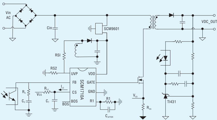
SCM1710A应用案例
