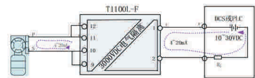
图9.无源系列信号调理模块应用接线之一
