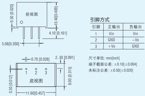
K78xxM-1000R3系列 LxWxH: 10.4x11.60x8.00(mm)
