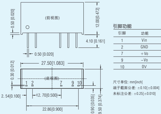
IE05_KS-1WR3系列 LxWxH: 27.50x9.50x12.00(mm)
