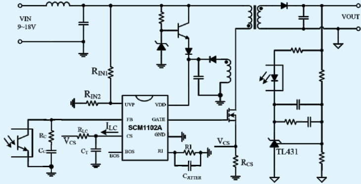
SCM1102A应用案例
