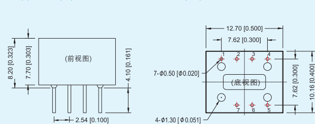
TD5(3)01MCAN(FD)系列 LxWxH: 12.70x10.16x7.70(mm)
