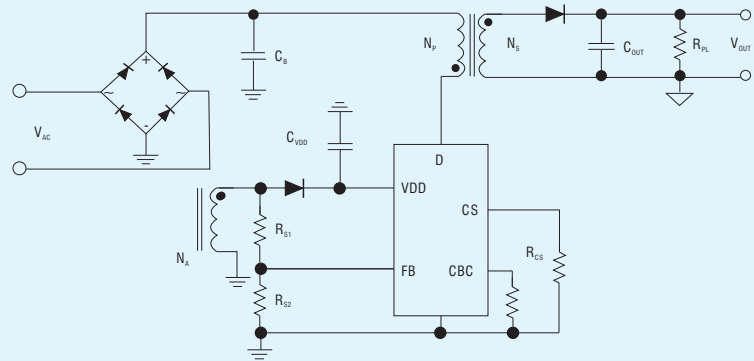
SCM1702A应用案例
