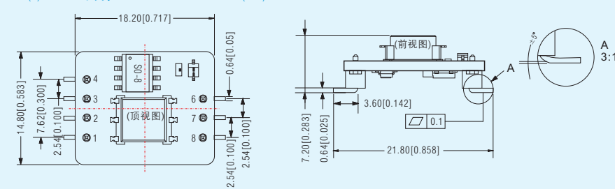
TD5(3)21SCANx系列: LxWxH: 18.20X14.80X7.20(mm)
