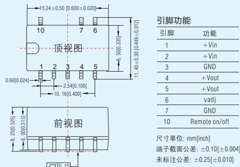
K78_T-500R3/K78_T-1000R3系列 LXWXH: 11.40X15.24X8.25(mm)
