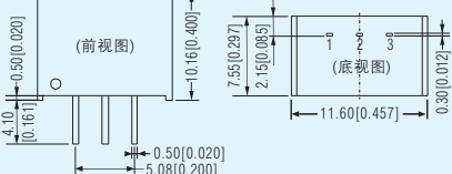
K78-500R3系列(灌封) LxWxH: 11.60x7.55x10.16(mm)
