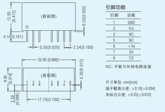
封装尺寸 LxWxH: 22.00x9.50x12.00(mm)
