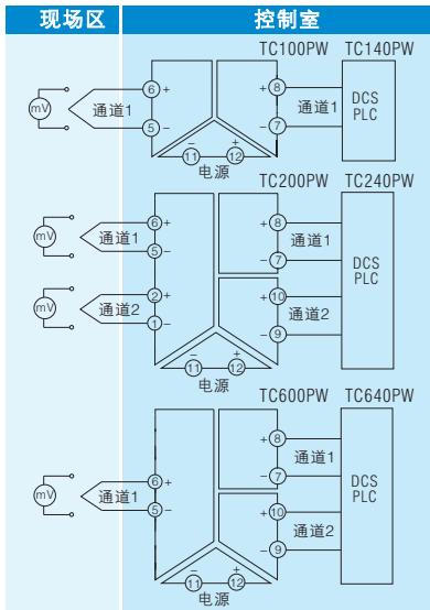
接线图
