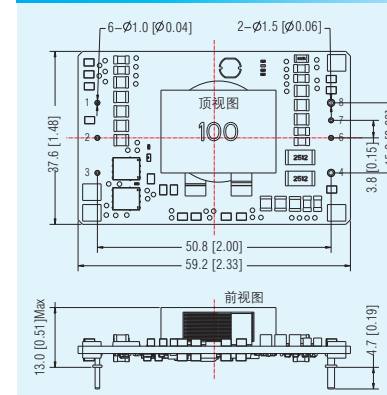
封装尺寸 LxWxH: 59.2x37.60x13.00(mm)
