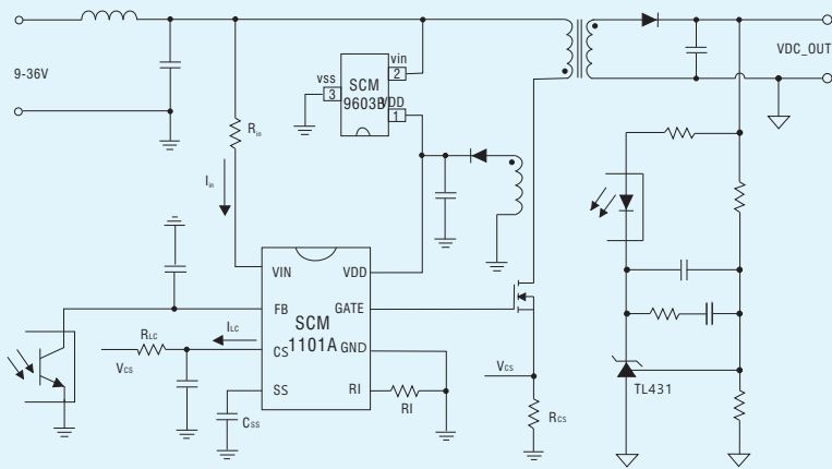
SCM1101A应用案例
