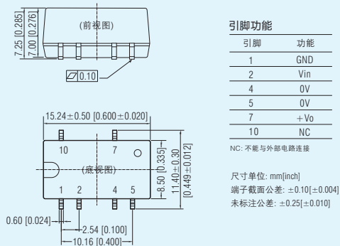
IF05_XT-1WR3系列 LxWxH: 15.24x11.20x7.25(mm)
