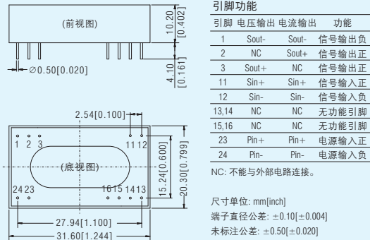
封装尺寸 LxWxH: 31.60x20.30x10.20(mm)
