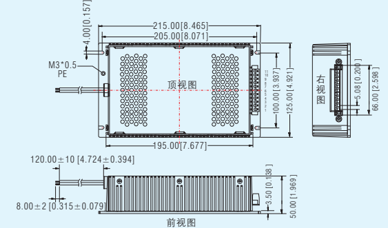
PV200-29Bxx系列 LxWxH: 215.00x125.00x50.00(mm)
