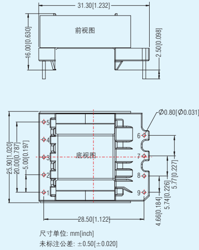
TTLHE25-20B-D 系列 LxWxH: 25.90x31.30x16.00(mm)
