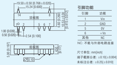
IF_RT-1W系列 LxWxH: 19.50x10.53x5.00(mm)
