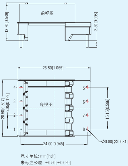
TTLHE20-20B-D 系列 LxWxH: 20.50x26.80x13.70(mm)
