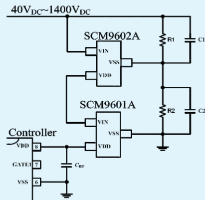
SCM9602A应用案例
