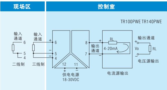
接线图
