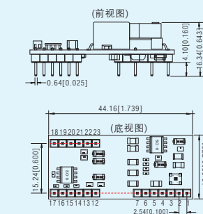
TLAxx-03K485/TLAxx-03K485L 系列: LxWxH: 44.16x19.62x12.24(mm)
