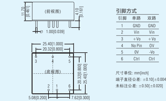
URA/B_YMD-10WR3、VRB_YMD-10WR3系列 LxWxH: 25.40x25.40x11.70(mm)
