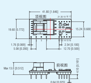
TLAxx-03KCAN 系列: LxWxH: 41.80x19.60x13.00(mm)
