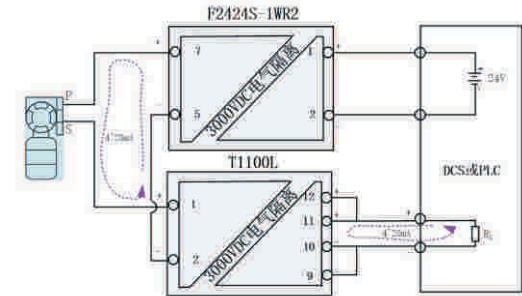
图10.无源系列信号调理模块应用接线之二
