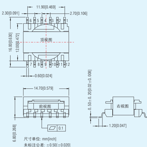
TTURB-20T 系列 LxWxH: 16.00x14.70x6.80(mm)
