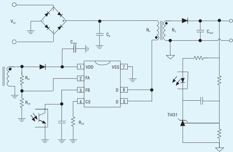
SCM1703A应用案例
