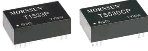
TxxxxP系列:LxWxH: 31.60x20.30x10.20(mm)
