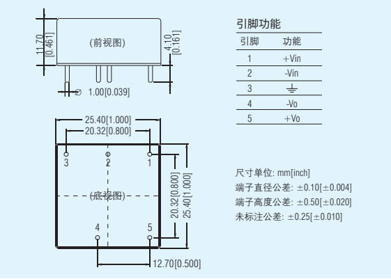
接线式A2S拓展封装
