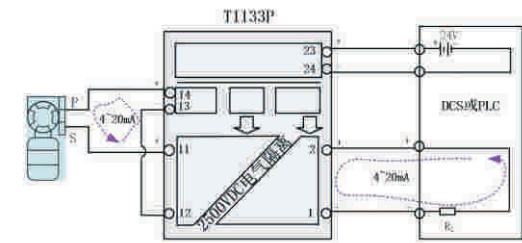
图11.有源系列信号调理模块应用接线之一
