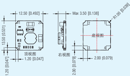
K78_JT-500R3系列 LxWxH: 27.50x9.50x12.00(mm)
