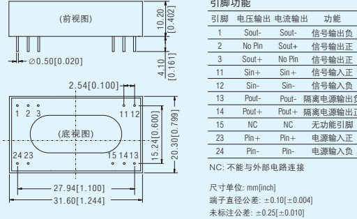
TxxxxCP系列:LxWxH: 31.60x20.30x10.20(mm)
