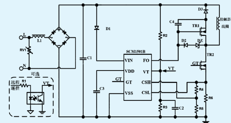
SCM1501B应用案例
