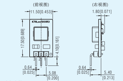
K78L-1000R3 系列(裸板) LxWxH: 11.50x7.20x17.50(mm)
