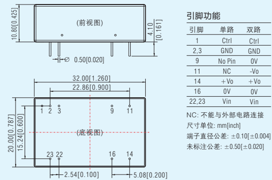
VRA/B_ZP-10WR3 & URA/B_ZP-10WR3系列 LxWxH: 32.00x20.00x10.80(mm)
