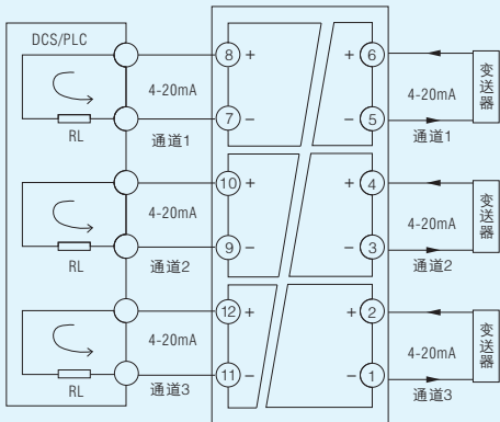
电流源应用接线图
