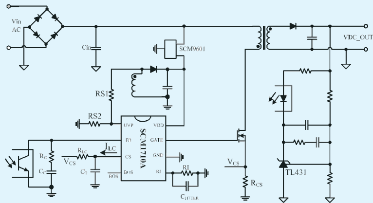
SCM9601A应用案例
