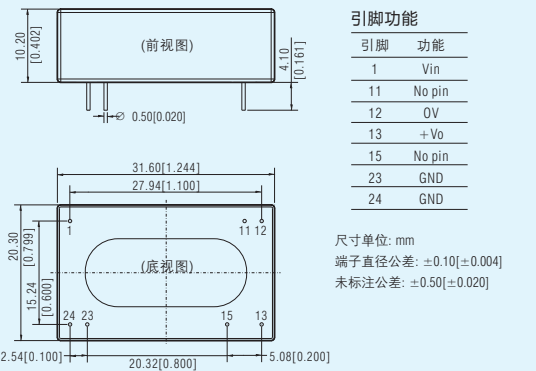
URH_P-6WR3系列 LxWxH: 31.60x20.30x10.20(mm)
