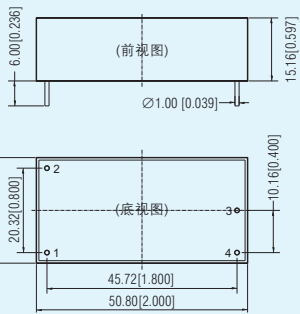
LD03系列: LxWxH: 50.80x25.40x15.16(mm)
