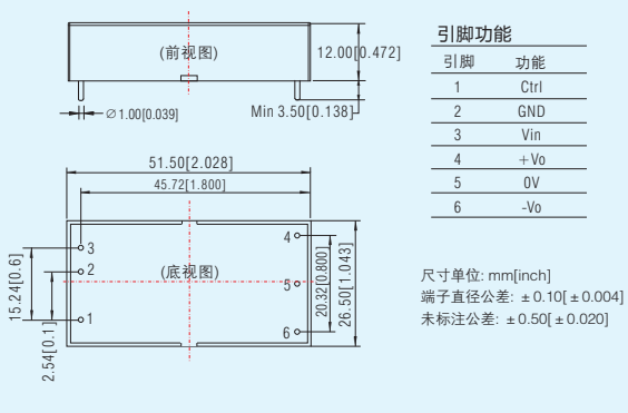
URH_LP-20WR3系列 LxWxH: 51.50x26.50x12.00(mm)
