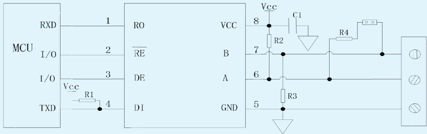
SCM3401A应用案例
