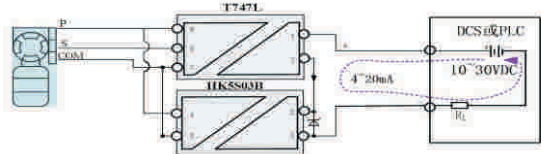
图13.两线制仪表接口模块应用接线
