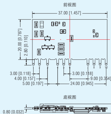
LSC15-26Mxx 系列: LxWxH: 37.00x20.00x4.60(mm)
