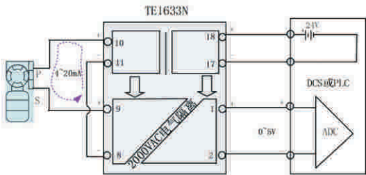
图12.有源系列信号调理模块应用接线之二
