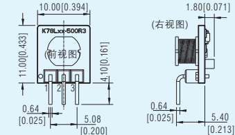
K78L-500R3系列(裸板) LxWxH: 10.00x7.20x11.00(mm)
