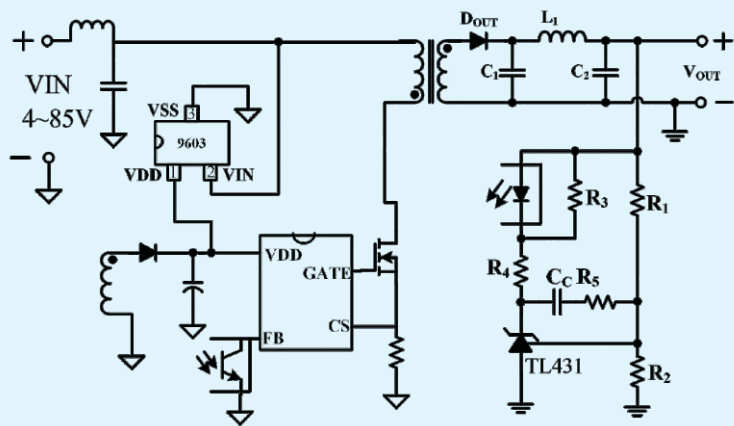
SCM9603B应用案例
